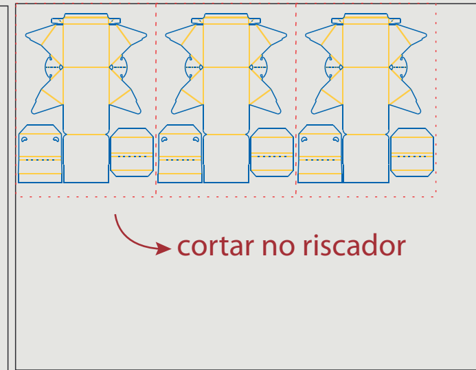
VOILA P PAPELÃO ONDA E 4/0 - 158x123cm
