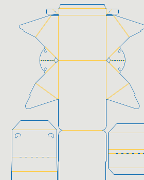
VOILA P ONDA E 4/0 - 46x57cm
