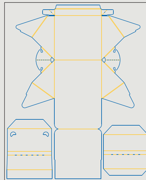
VOILA M ONDA E 4/0 - 62x76cm
