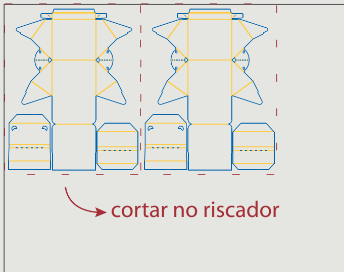
VOILA M PAPELÃO ONDA E 4/0 - 158x123cm
