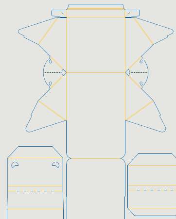
VOILA M ONDA E 4/0 - 60x74cm
