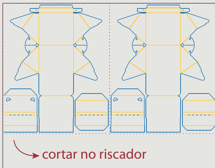
VOILA G PAPELÃO ONDA E 4/0 - 158x123cm
